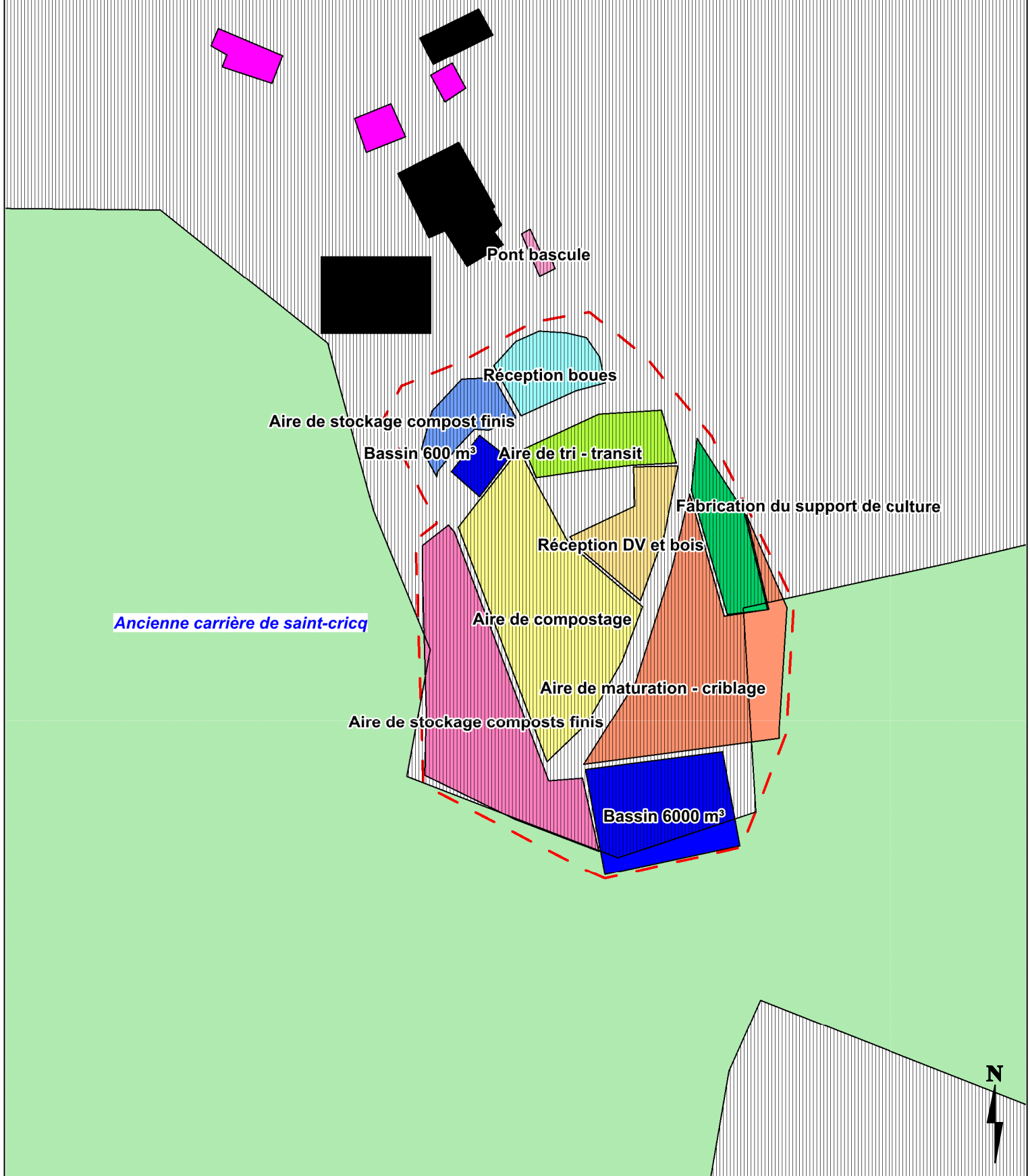
- Plan d'ensemble et des abords de l'installation -
