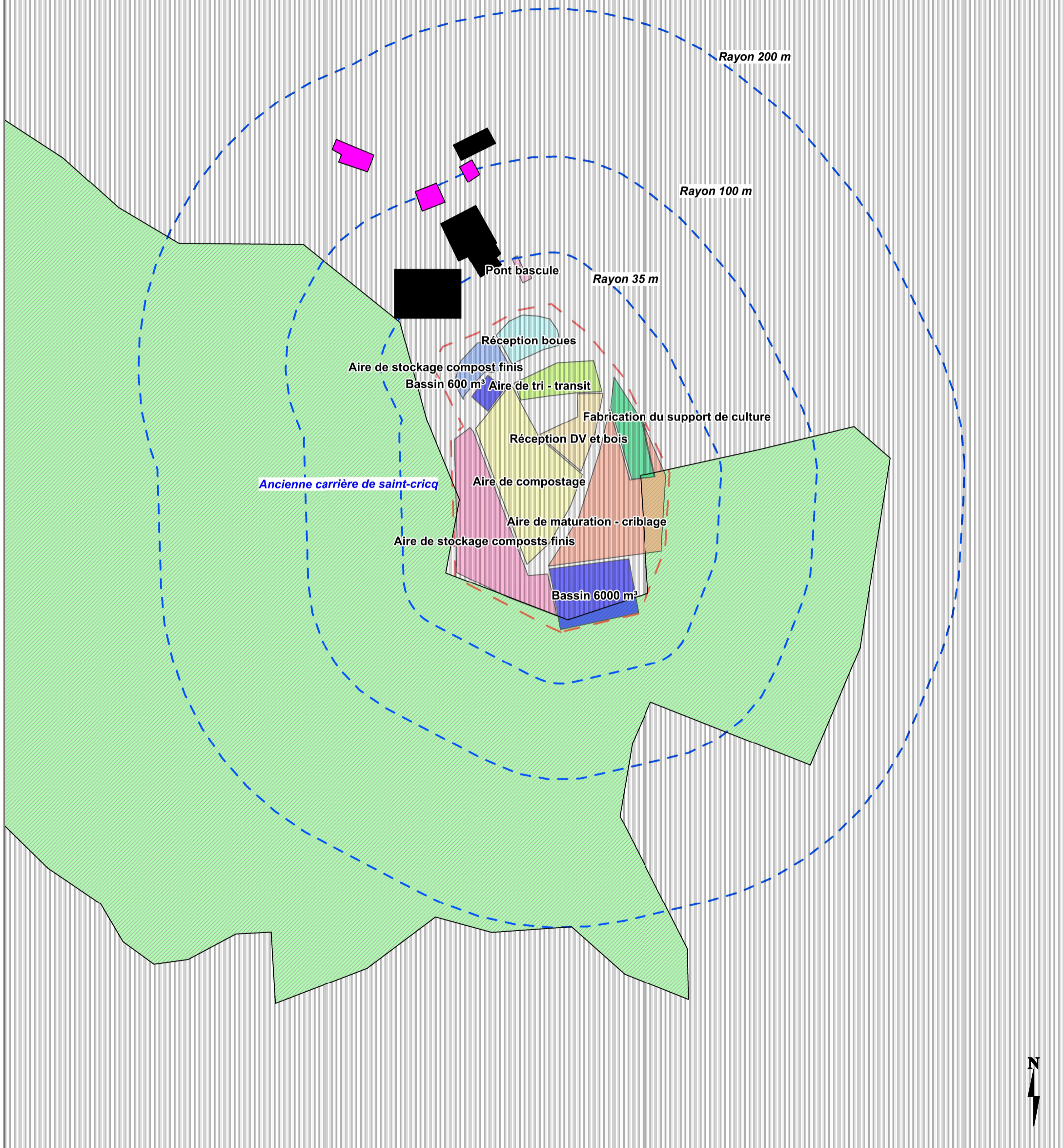
- Plan d'ensemble et des abords de l'installation -
